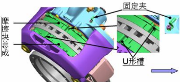
图 4-7：摩擦块总成装入托架
