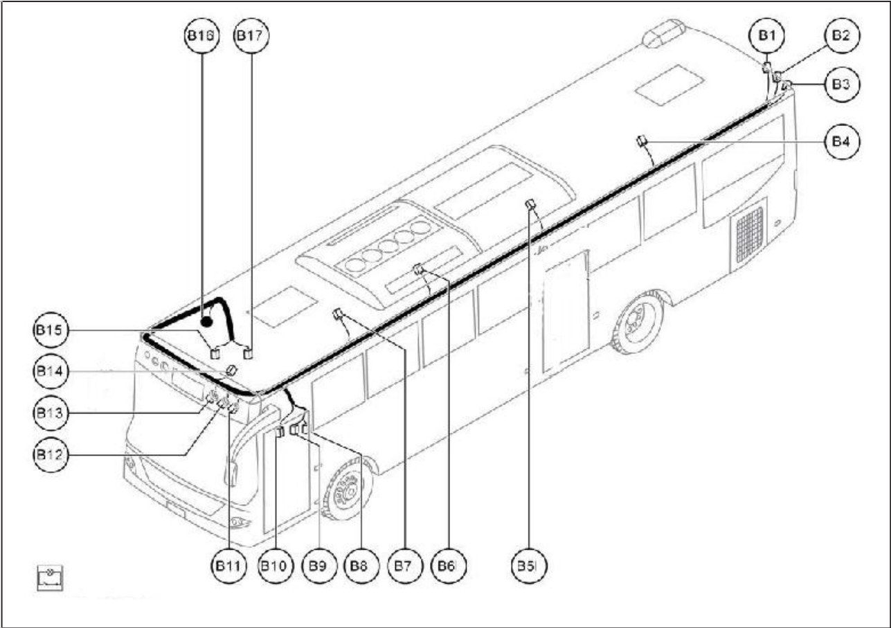
右顶架线束连接示意图
