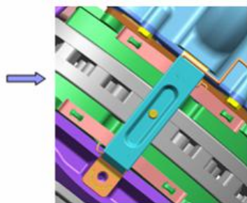
图 4-9：装入弧形压条
