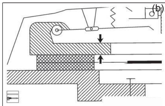
(b). 检查离合器压盘的厚度。
