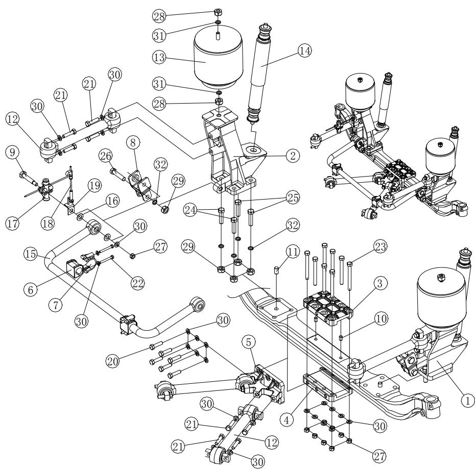
DWG09F 前悬结构示意图:
