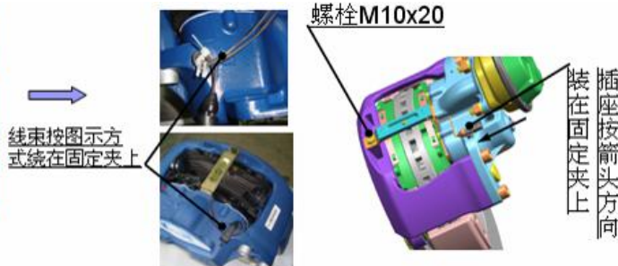
图 4-10：绕线束、装螺栓 M10x20、制动块压板
