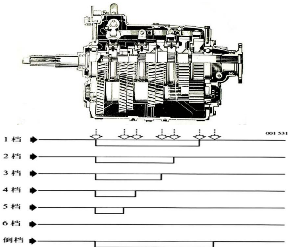
变速器各挡传动路线
